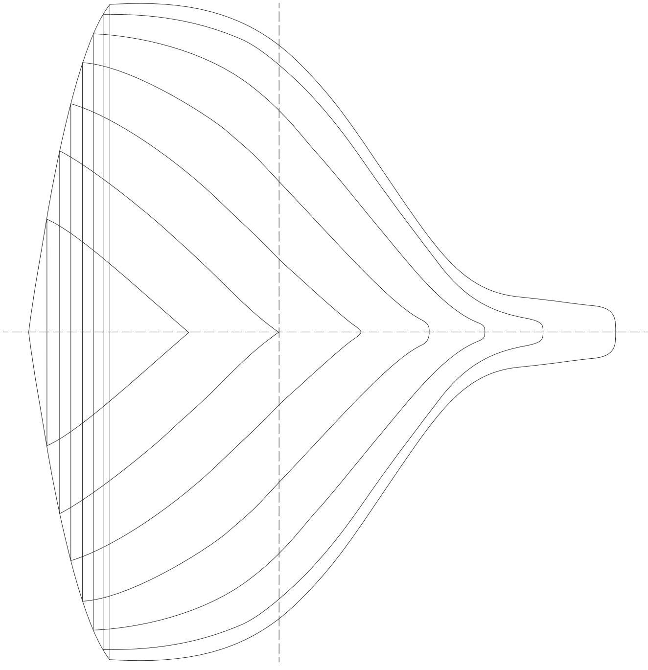
PLAN DE FORME AVANT 1/25
